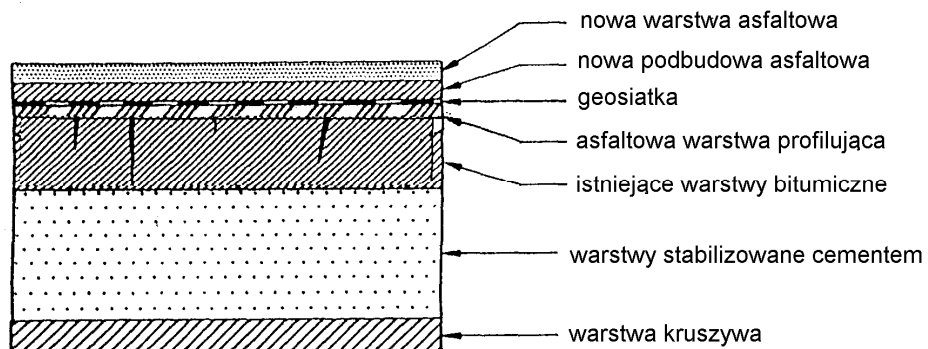
Rys. 3. Wzmocnienie nawierzchni asfaltowej na podbudowie z gruntu stabilizowanego cementem
