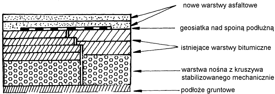
Rys. 2. Wzmocnienie nawierzchni asfaltowej w strefie poszerzenia nawierzchni
