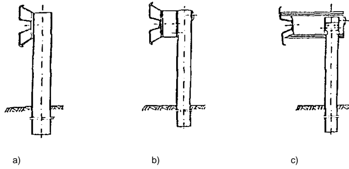
Załącznik 11.3. Zasady określania wysokości prowadnicy bariery nad poziomem terenu, wg [32]
