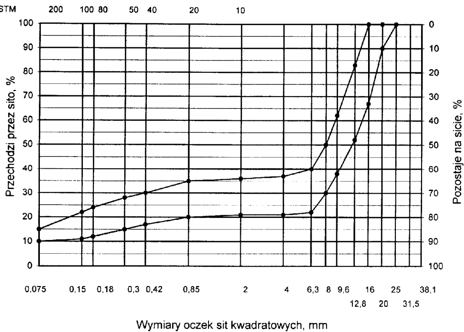
Rys. 5. Krzywe graniczne uziarnienia mieszanki mineralnej BA od 0 do 20 mm (mieszanka o nieciągniętym uziarnieniu) do warstwy ścieralnej nawierzchni drogi o obciążeniu ruchem od KR3 do KR6
