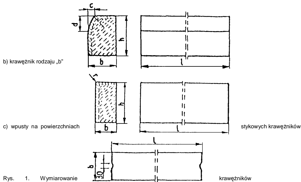
Rys. 1. Wymiarowanie krawężników
