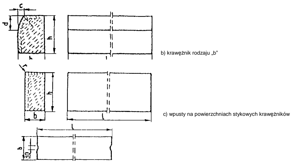
Rys. 1. Wymiarowanie krawężników
