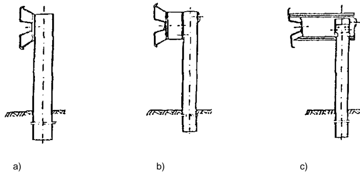
Załącznik 11.3. Zasady określania wysokości prowadnicy bariery nad poziomem terenu, wg [32]
