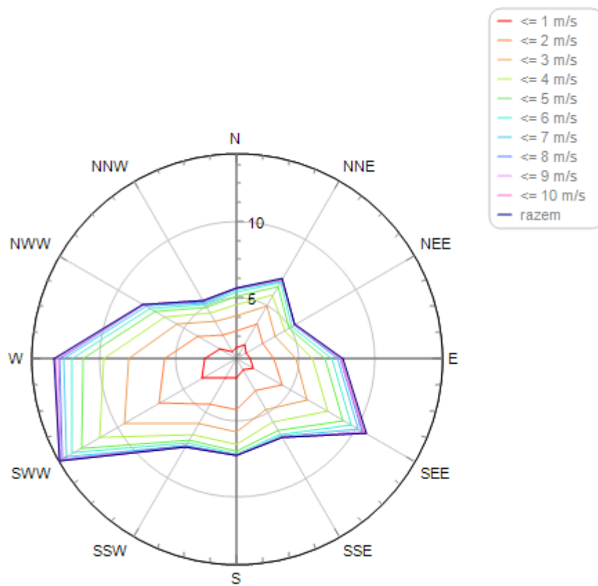
Rycina 7. Róża wiatrów dla stacji w Toruniu
