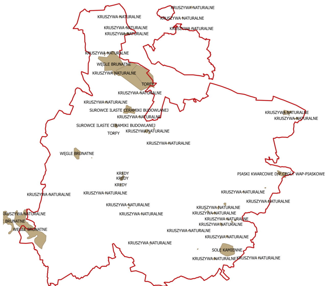
Rycina 19. Rozmieszczenie złóż geologicznych na terenie powiatu włocławskiego
