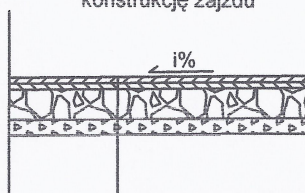
Przekrój przez konstrukcję zjazdu
